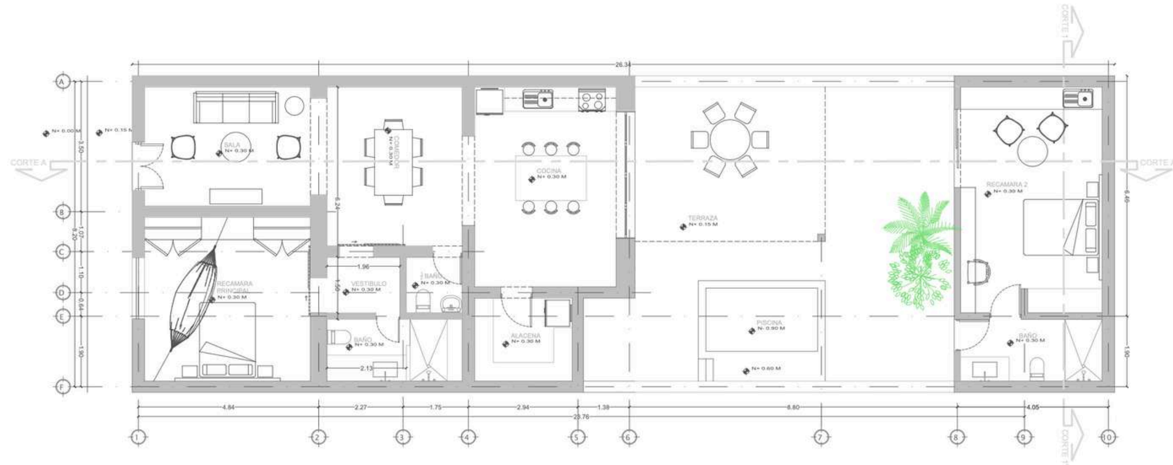
PLANTA BAJA DE PROYECTO ESC. 1:75
